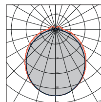
Ottica 113°
